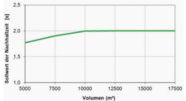
Darstellung der Nachhallzeitsollwerte für Sporthallen in Abhängigkeit vom Raumvolumen
